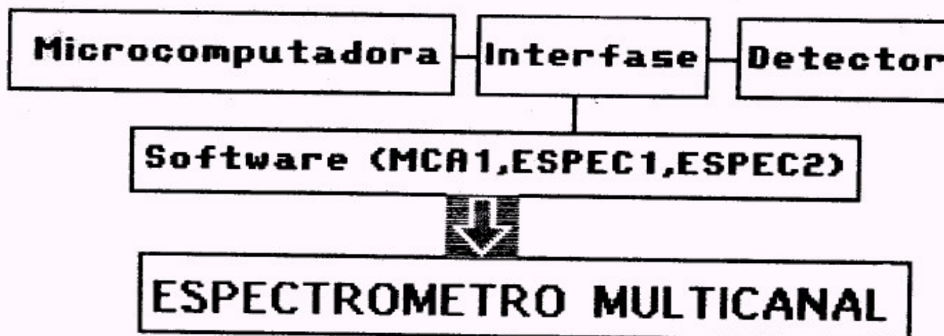
Figura 1. Diagrama de bloques del sistema para la adquisición, operaciones fundamentales y procesamiento analítico de espectros de radiación gamma.
