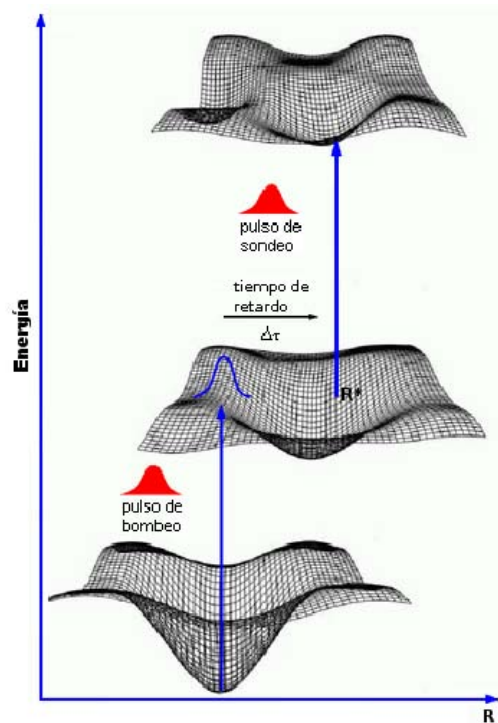
Figura 1. Representación esquemática de la técnica de bombeo-sonda. El pulso de sonda, retrasado un intervalo de tiempo \Delta\tau con respecto al pulso de bombeo, promueve el paquete de ondas al estado excitado 2. La fluorescencia desde este último estado es la señal que se mide en el experimento.
